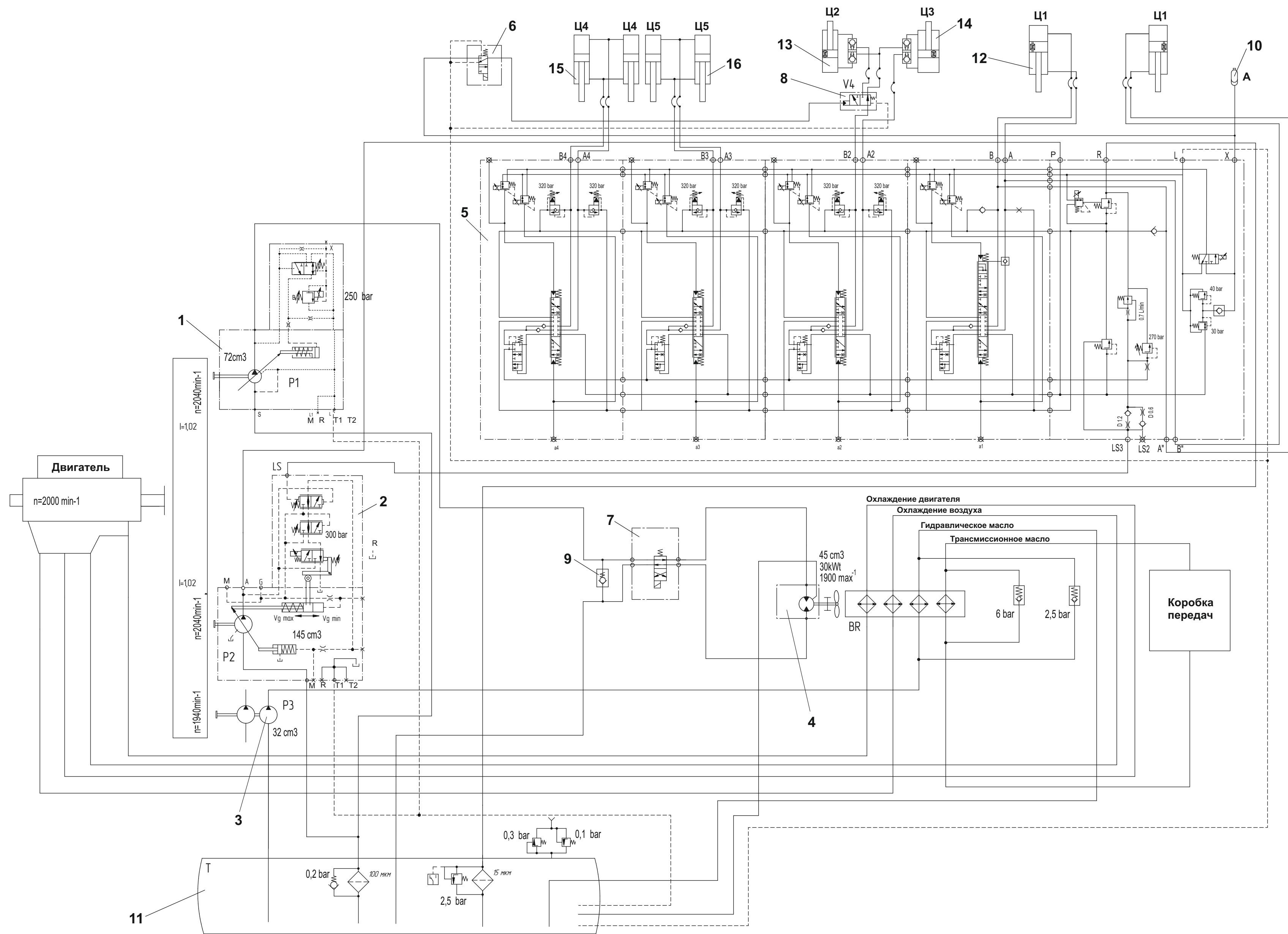
Схема принципиальная гидравлическая навесного оборудования и привода вентилятора на бульдозер Т-30.03К/ К2
