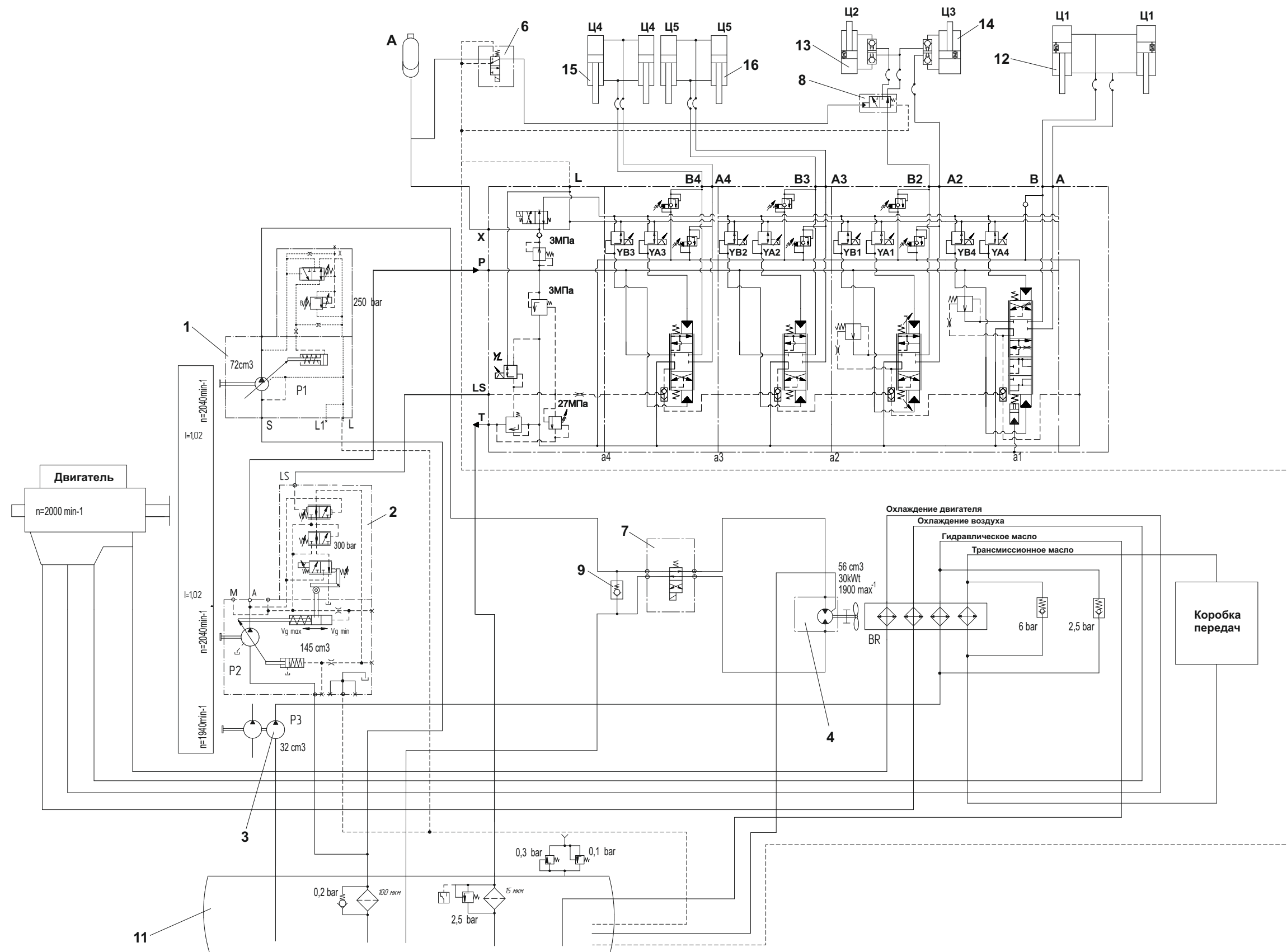
Схема принципиальная гидравлическая навесного оборудования и привода вентилятора на бульдозер Т-30.03Т/Т2
